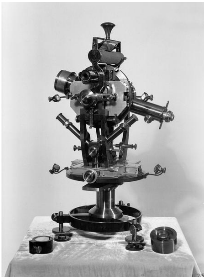
Theodolit. Fotografie, Beilage zur Patentschrift von 1907 (Bundesamt für Landestopografie). [...]
